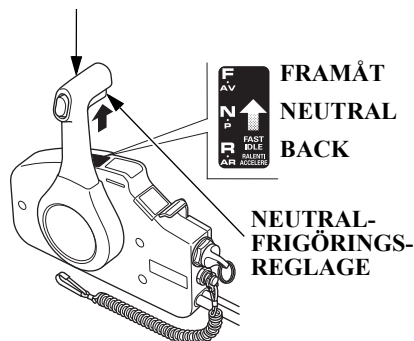
FJÄRREGLAGESPAK
