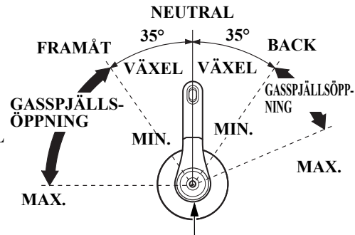
FJÄRRKONTROLLSPAK
