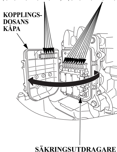
SÄKRINGSUTDRAGARE
