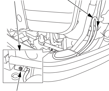
AVTAPPNINGSPLOGG
